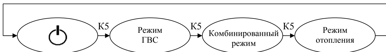
Рис. 5. Последовательность смены режимов работы котла
