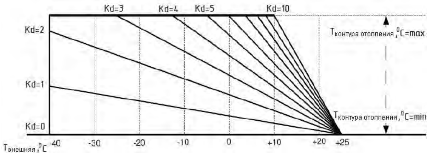
Рис. 6. График зависимости температуры в контуре отопления от внешней температуры
