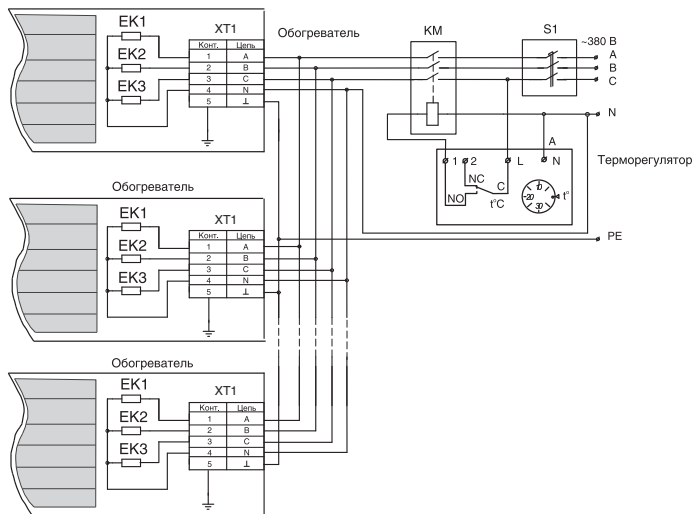
Рис. 2. Обогреватели VIN-3.0 и VIN-4.0
