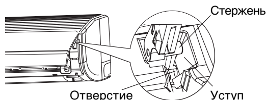
Установка передней крышки
