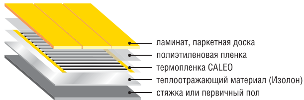
Рис. 27. Схема монтажа теплого пола CALEO под ламинат или паркетную доску
