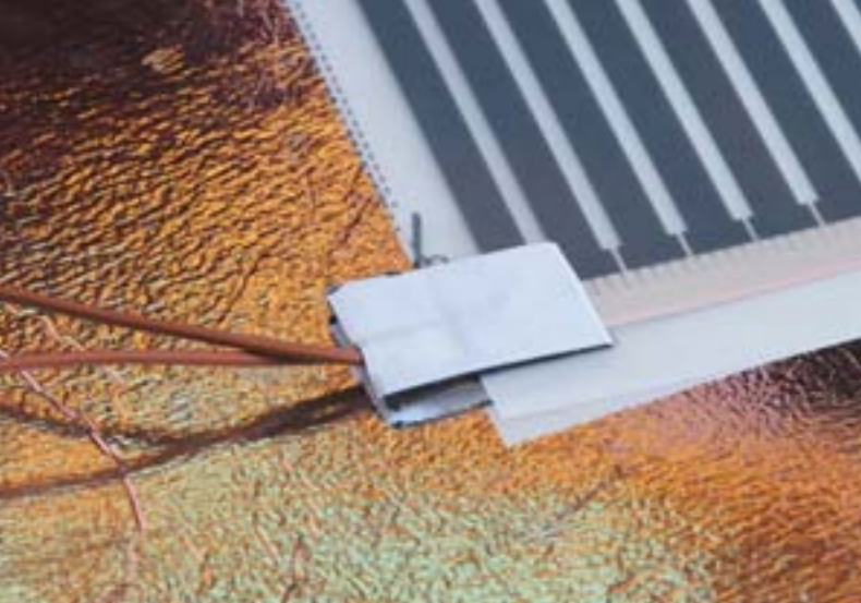
Рис. 19. Вид заизолированного контактного зажима с подключенными проводами
