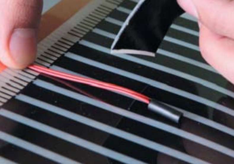
Рис. 23. Датчик прикрепляется к термолентке битумной изоляцией
