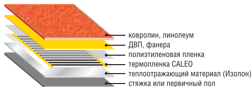
Рис. 3. Схема монтажа теплого пола CALEO под ковровин или линолеум
