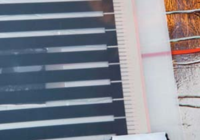
Рис. 25. Установленный и приклеенный датчик температуры пола. Вид сверху термопленки
