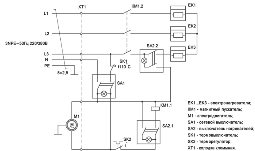
Рис.1. Схема электрическая
