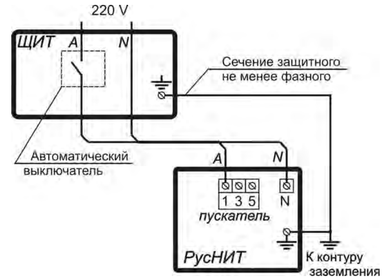
Рис.6. Схема подключения РусНИТ-205НМ,206НМ, 207НМ, 208НМ, 209НМ к однофазной сети .
