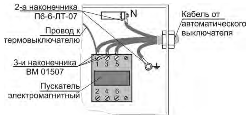
Рис.5. Подключение РусНИТ-206НМ, 207НМ, 208НМ, 209НМ к трёхфазной сети.
