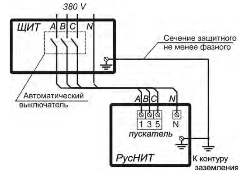
Рис.7. Схема подключения РусНИТ-206НМ, 207НМ, 208НМ, 209НМ к трёхфазной сети.
