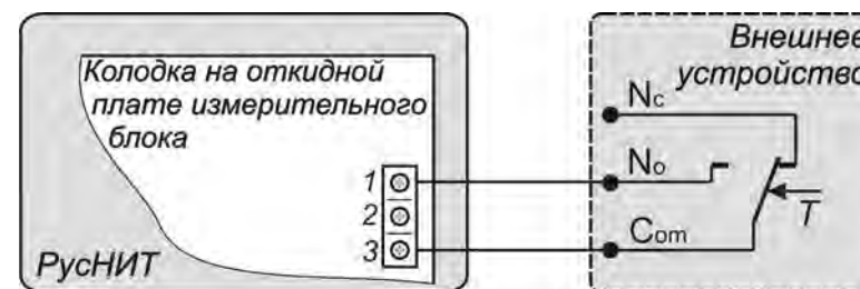
Рис.8. Подключение внешнего управляющего устройства.
