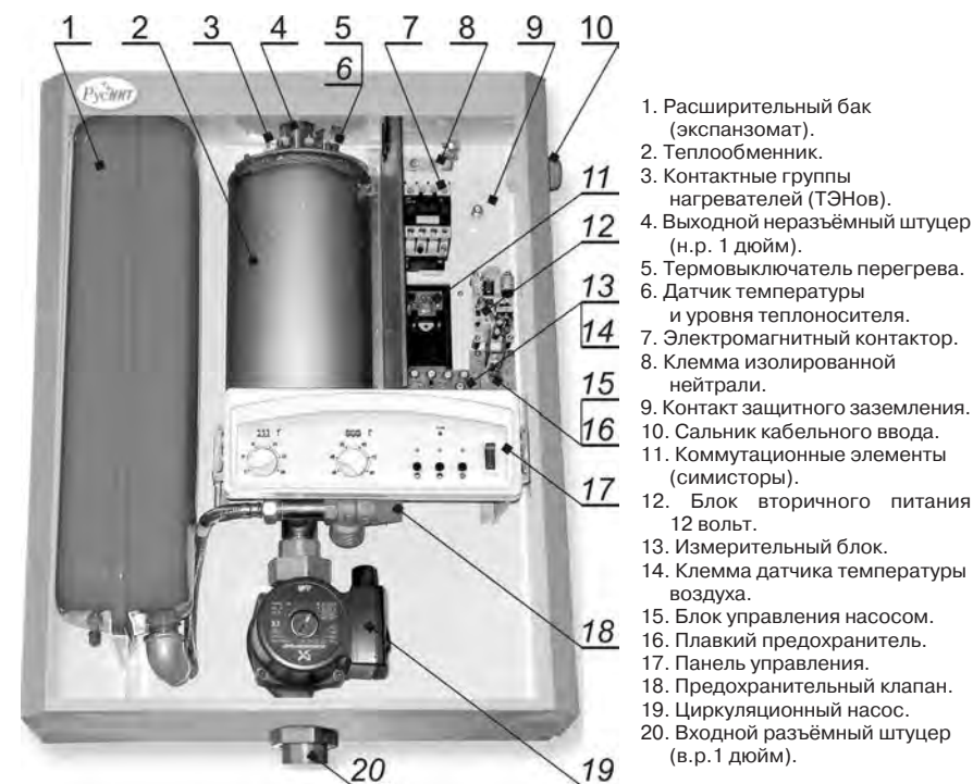
Рис.1. Состав отопителя.
