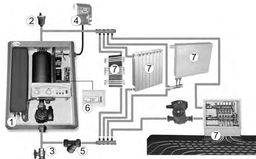
1. Отопитель. 2. Воздухоотводный клапан. 3. Вентиль. 4.Автоматический выключатель электросети. 5. Фильтр. 6. Внешнее регулирующее устройство. 7. Тепловые приборы Рис.3. Рекомендуемая схема монтажа отопительной системы.
