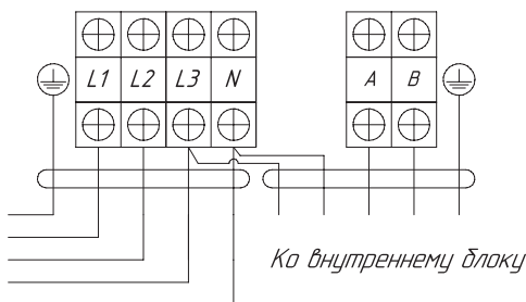
К электропитанию
