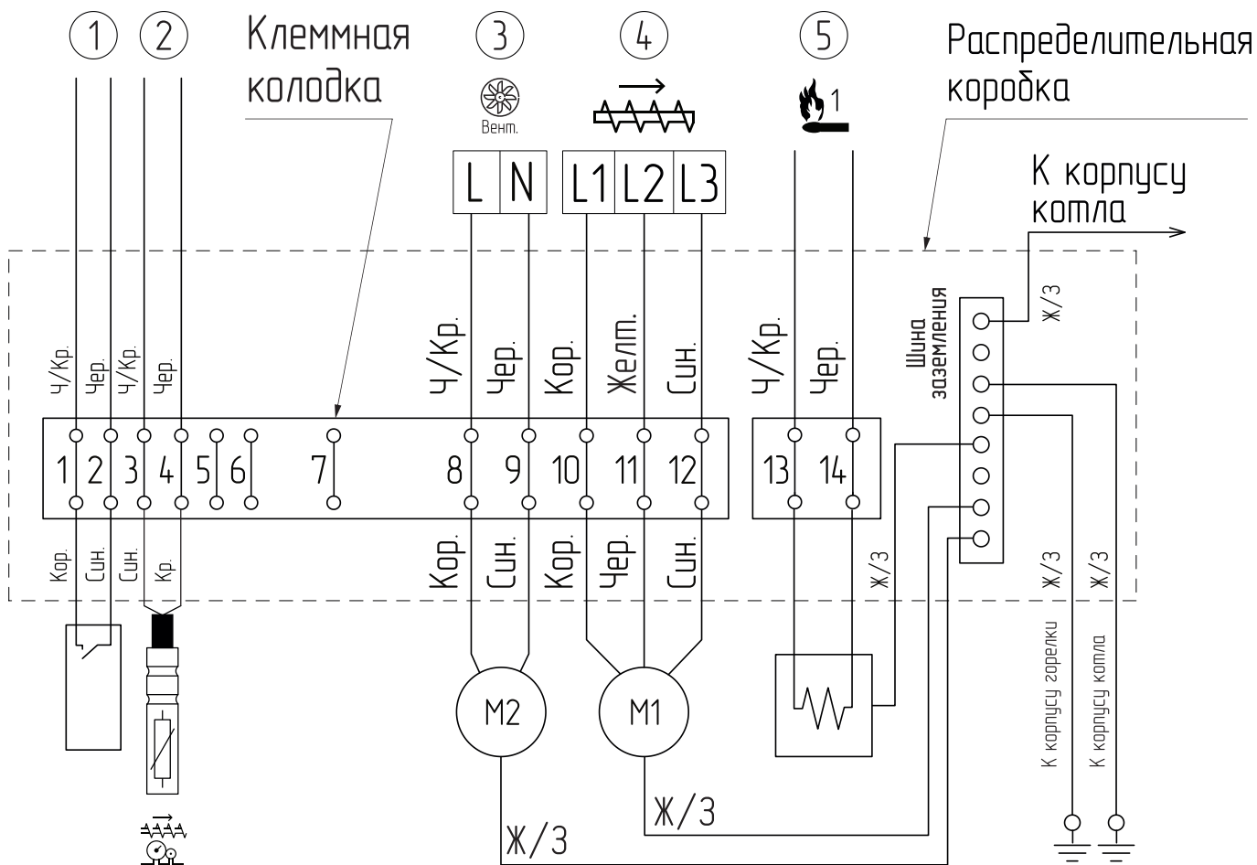
Рис.6 Схема распределительной коробки контроллеров ZOTA серии I-Line 223SFA для котлов ZOTA Stahanov 16-65 кВт
