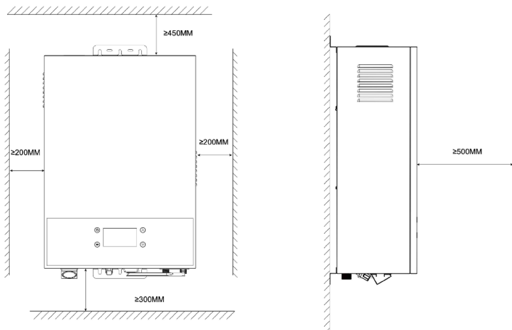
Рис. 5. Минимальные расстояния от электрического котла до поверхностей.
