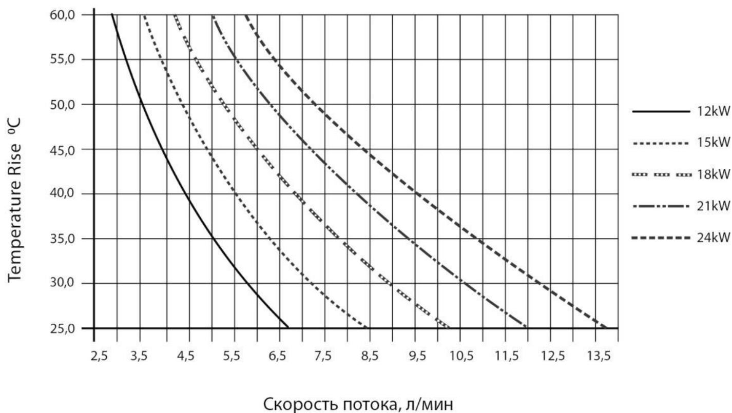
Рис. 4. График производительности системы ГВС
