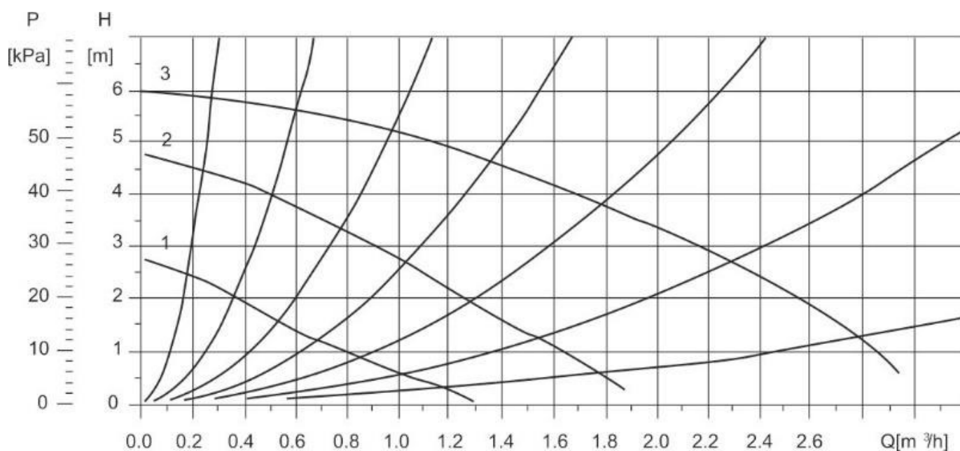
Рис. 15. Кривая характеристик давления насоса
