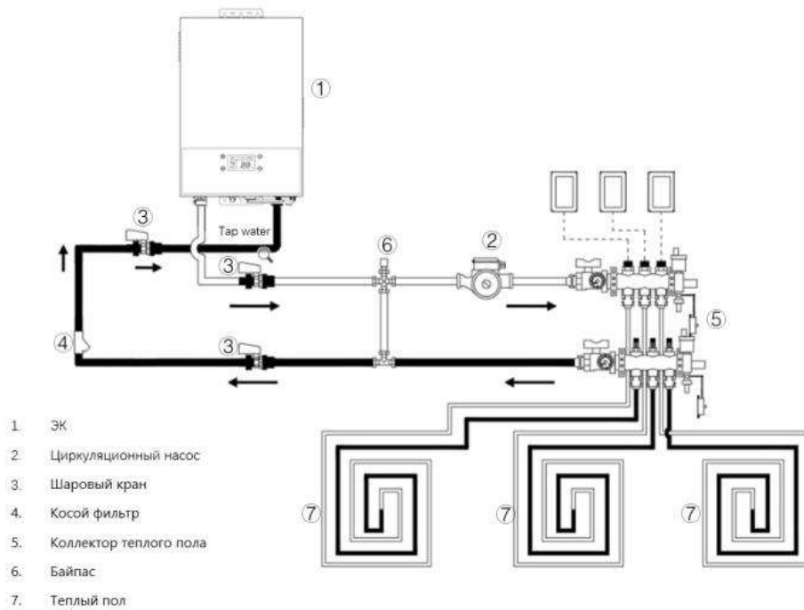
Рис. 8. Схема подключения «теплый пол + ЭК»
