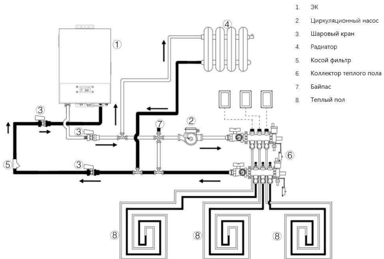
Рис. 8. Схема подключения «теплый пол + ЭК»
