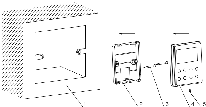
Схема установки проводного пульта
