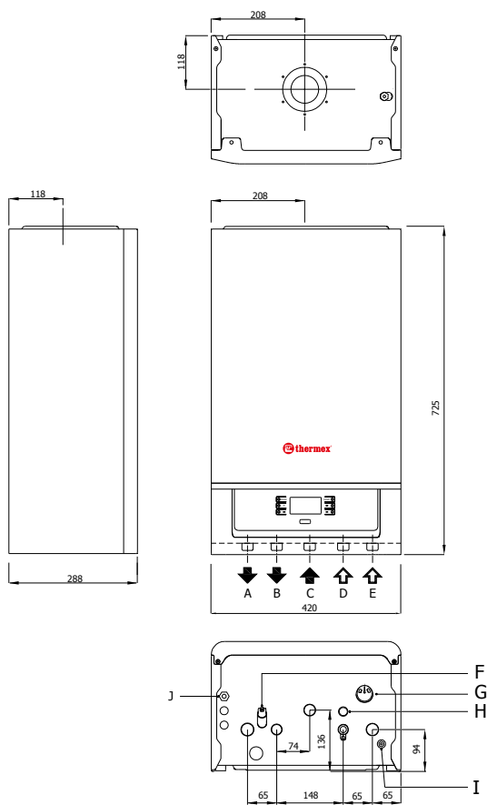
Рисунок 7. Размеры и подключения котла XantusPlus
