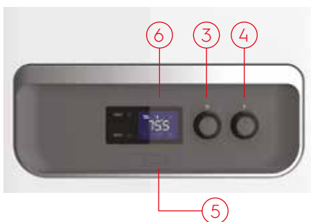
Рисунок 26 Автоматическая панель управления XANTUS
