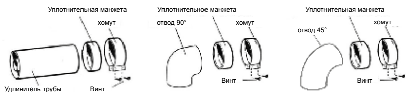
Рисунок 13. Монтаж элементов дымохода
