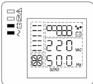
Рисунок 9 — состояние ЖК-дисплея и индикаторов в режиме «РЕЗЕРВ»
