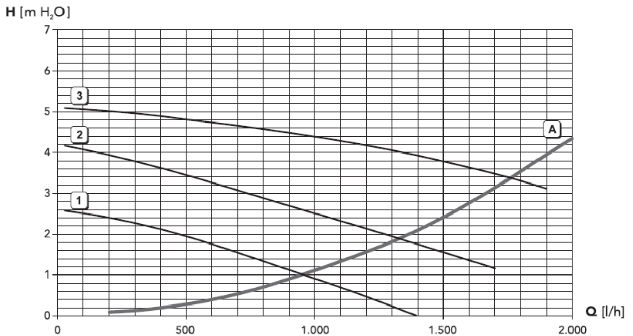
Рис. 12. Потери напора циркуляционных насосов. A – потери напора в котле; 1, 2 и 3 – скорость циркуляционного насоса
