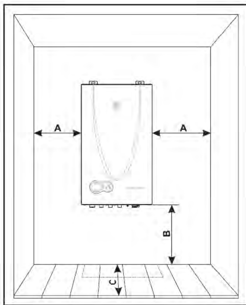
Рис. 5 Размещение котла.
