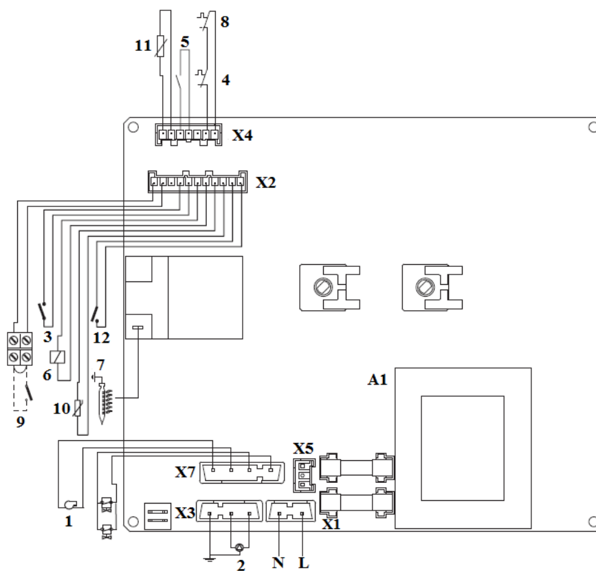
Рис.9. Принципиальная электрическая схема
