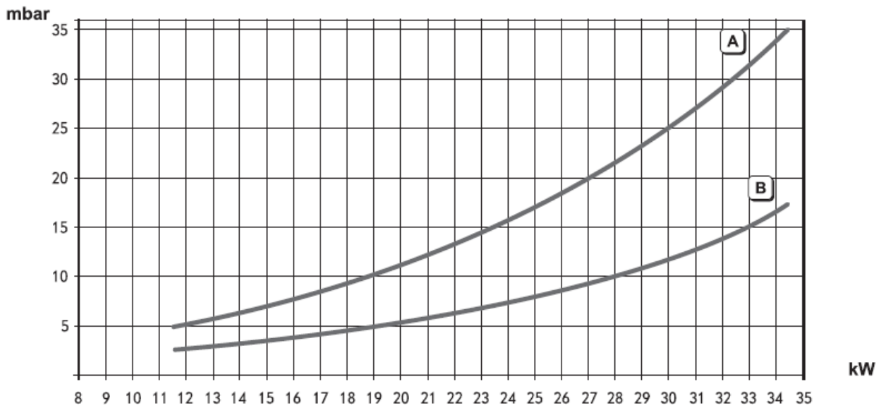
Рис. 13. График зависимости мощности котла от входного давления газа. A – сжиженный газ, B – природный газ.
