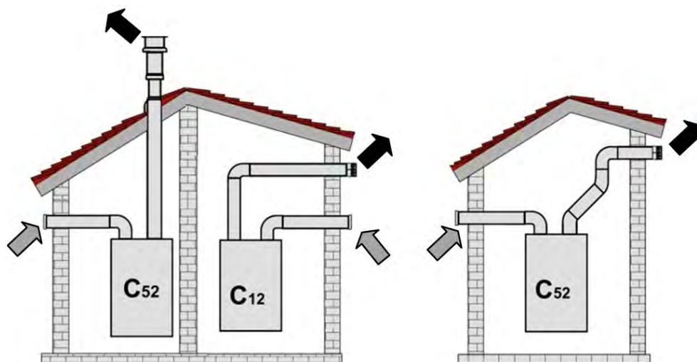
Рис. 16. Примеры систем дымоудаления собранных с помощью раздельных труб. Серой стрелкой обозначен приток воздуха, чёрной стрелкой поток продуктов сгорания
