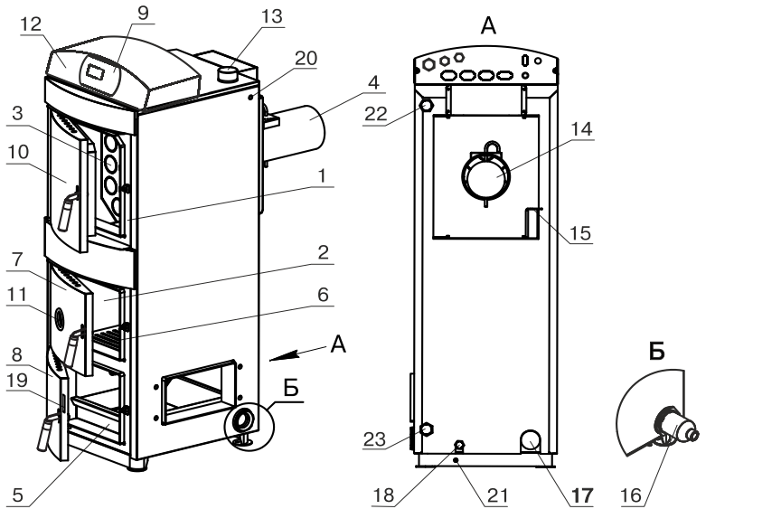
Рис.1 Котел пеллетный в сборе
